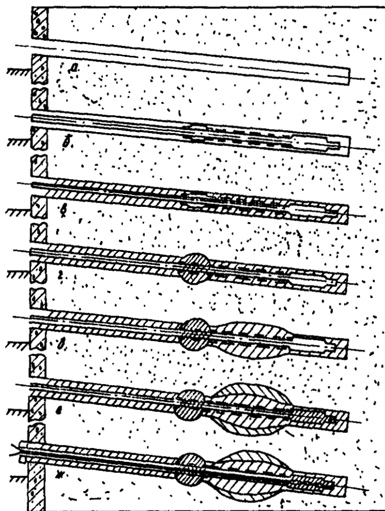
Черт. 17. Технологическая последовательность устройства постоянного анкера с манжетной трубой при внутреннем расположении тяги из канатной арматуры
