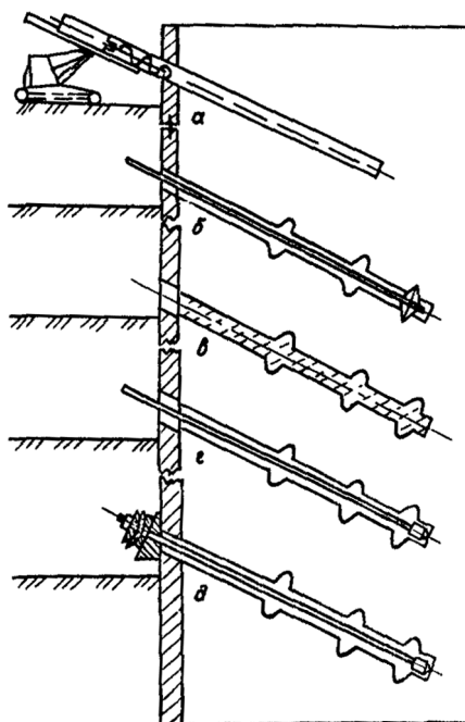
Черт. 14. Технологическая последовательность устройства анкера в связных грунтах с разбуhrиванием ушщрений
