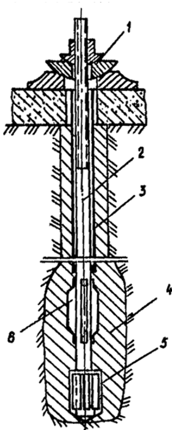
Черт. 4. Временный анкер со стержневой арматурой.
