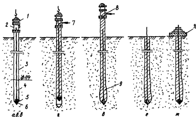
Черт. 15. Технологическая последовательность устройства вертикального анкера с вибропогружателем
