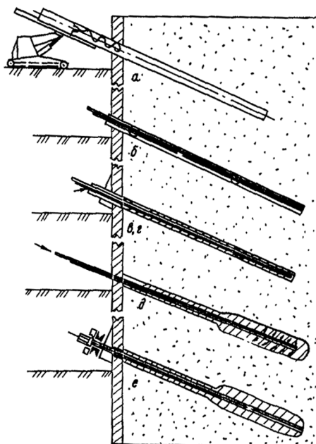
Черт. 13. Технологическая последовательность устройства анкера с применением инъекционной трубки
