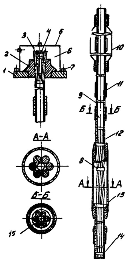
Черт. 9. Постоянный инъекционный анкер с манжетной трубой при внутреннем расположении анкерной тяги из канатной арматуры
