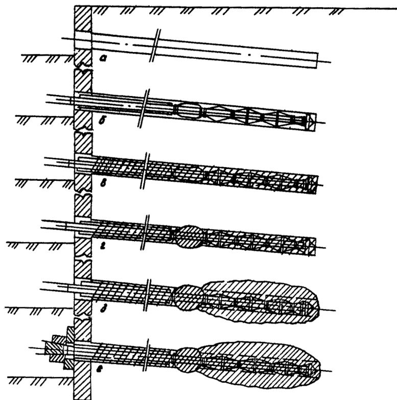
Черт. 16. Технология устройства временного инъекционного анкера с манжетной трубой при наружном расположении тяги из канатной арматуры
